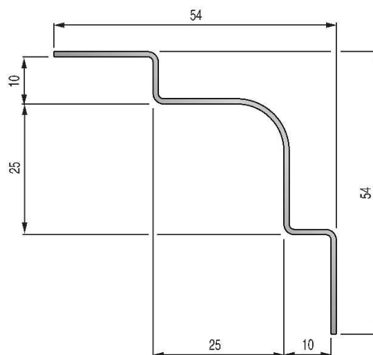
Modèle pour angle rentrant
