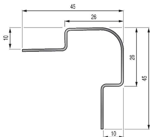
Modèle pour angle sortant
